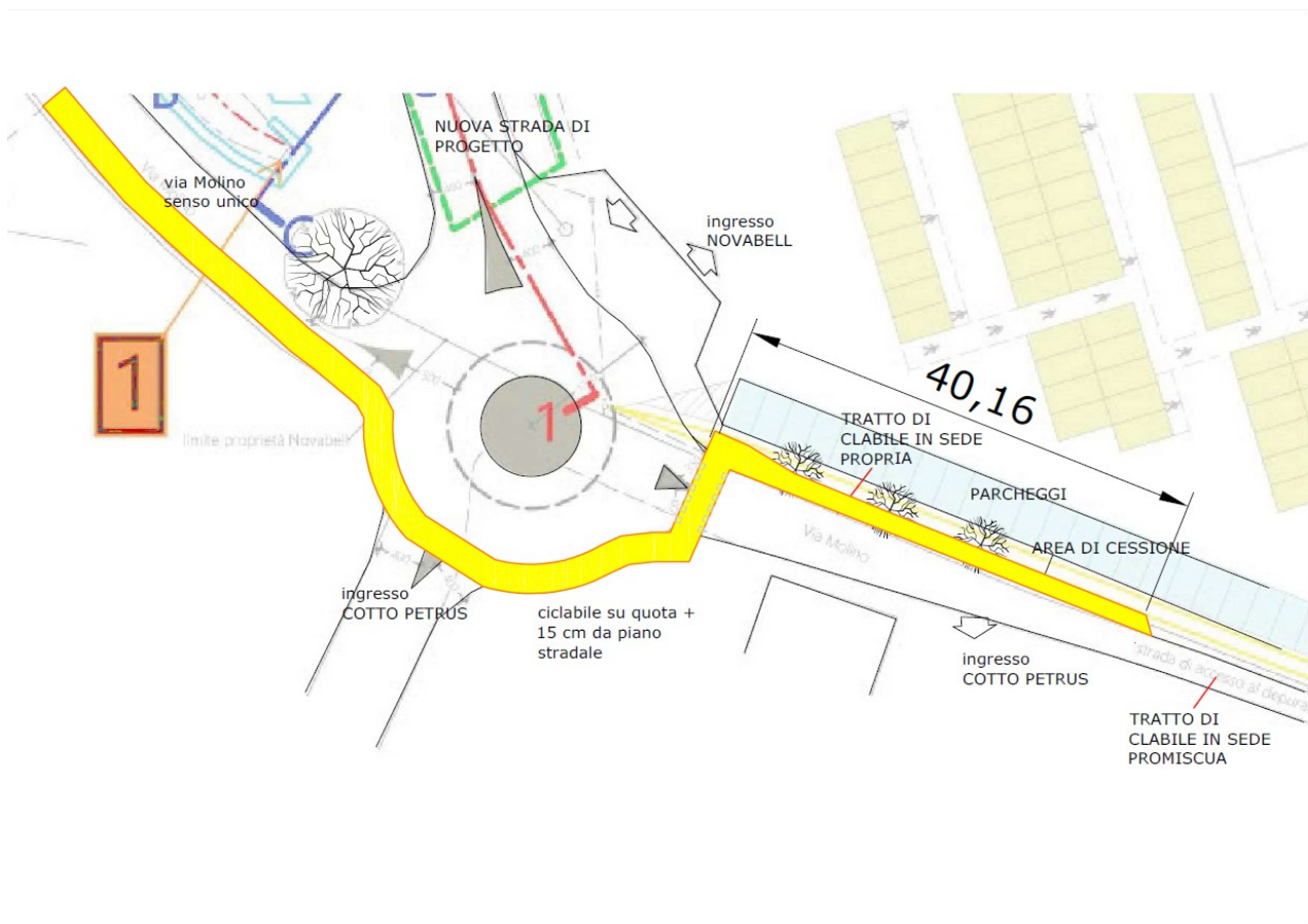
Schema grafico della rotatoria con ipotesi pista ciclabile
