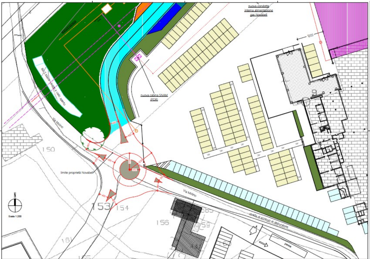
Schema grafico della rotatoria
